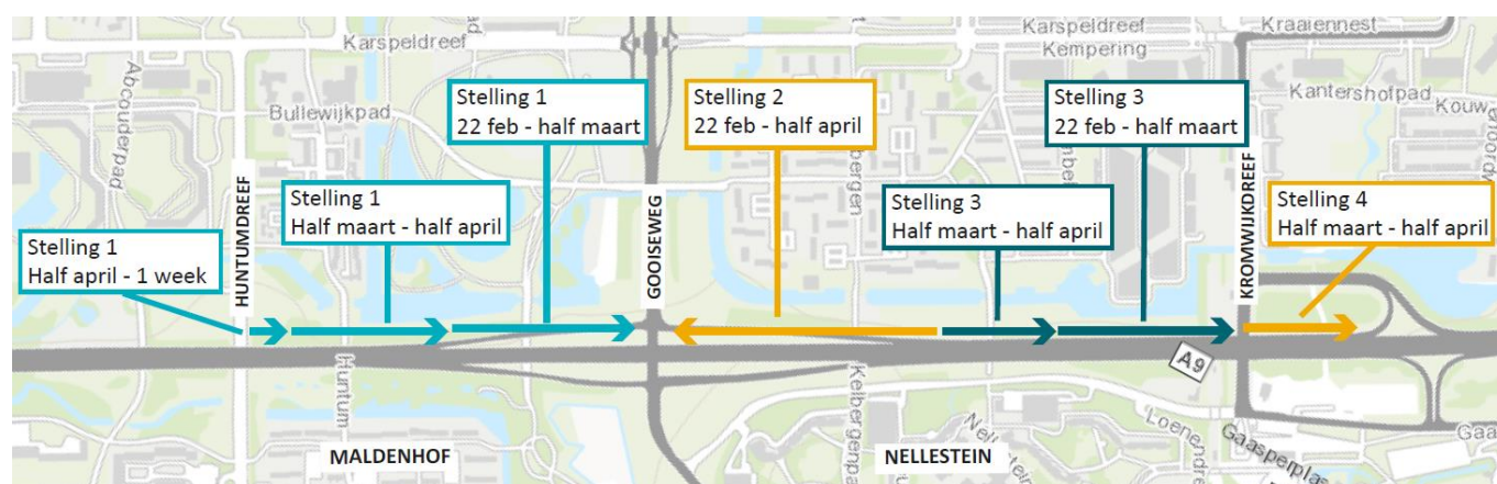
Afbeelding: de planning van het aanbrengen van de heipalen.
