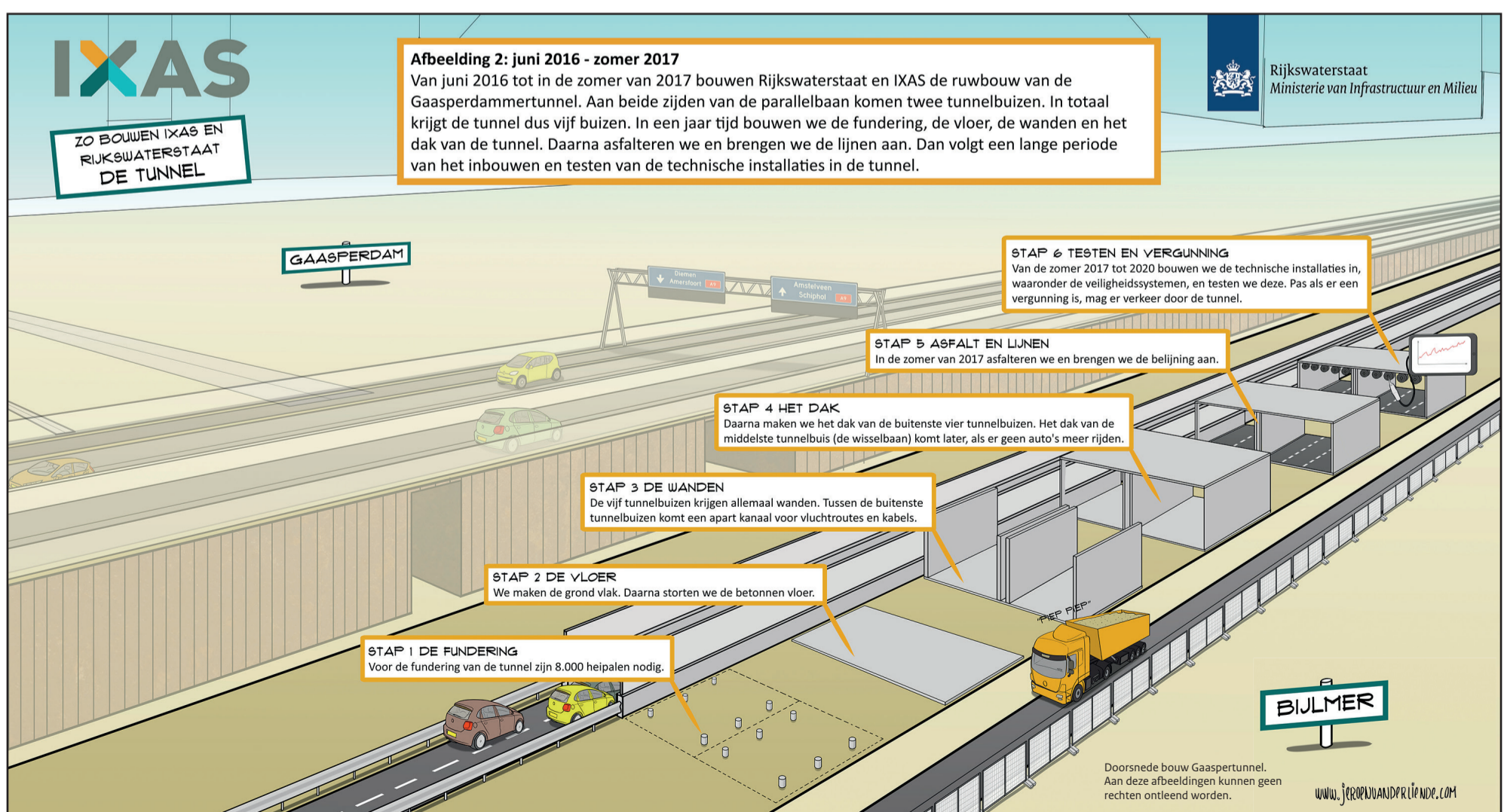
De bouwstappen van de tunnel in beeld
