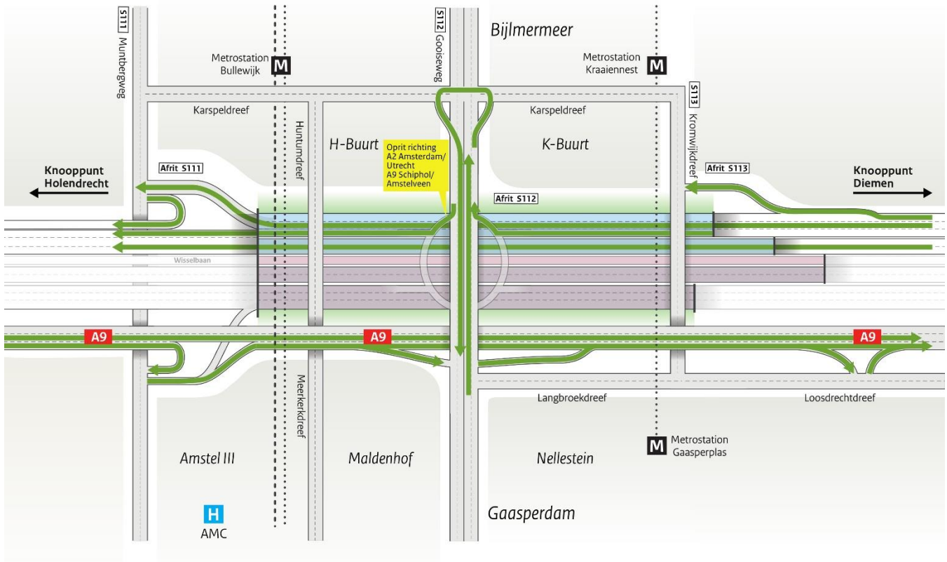
Afbeelding 2 Verkeerssituatie A9 Gaasperdammerweg vanaf maandag 24 augustus 05:00 uur
