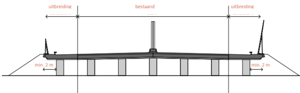
Dwarsdoorsnede uitbreiding
