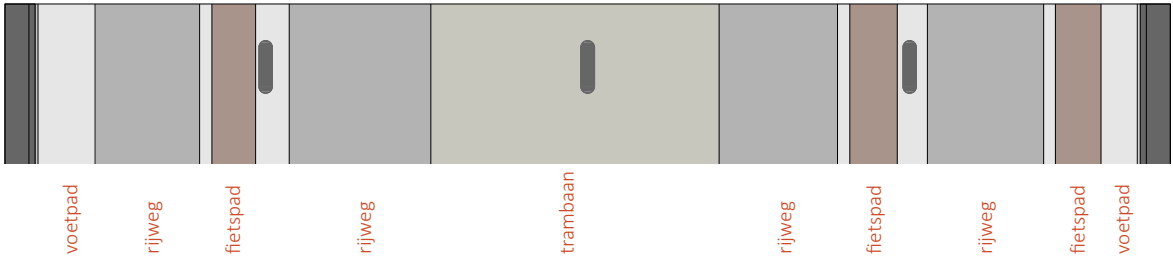
Profiel inrichting onderdoorgang
